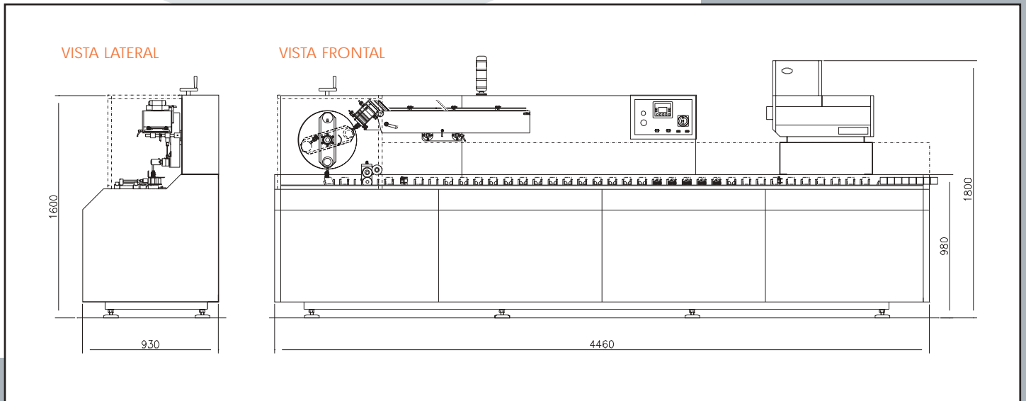
Innovador cabezal rotativo de carga de estuches con válvula mecánica de vacío. Estabilidad en alta velocidad.
